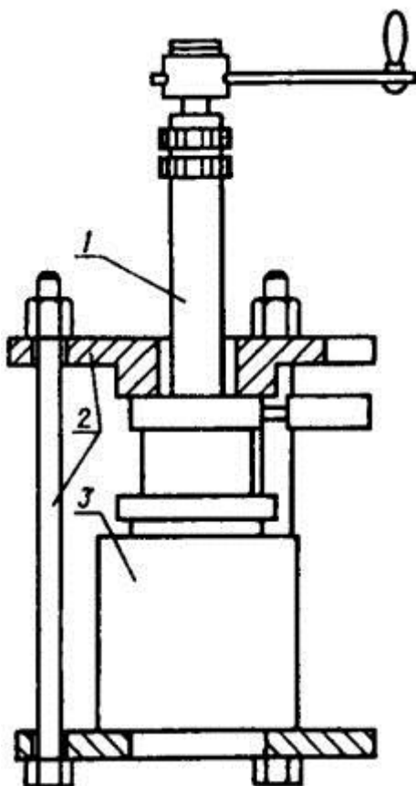
1 - фильтратометр; 2 - крепежное устройство; 3 - бетонный образец
